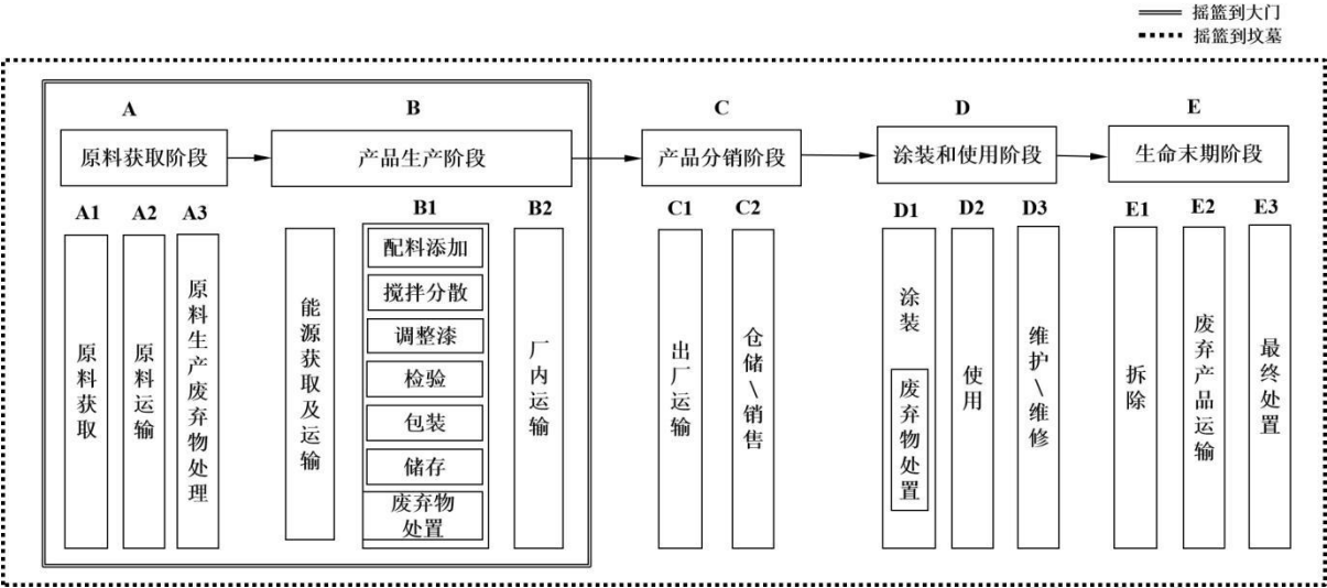
图 1 集装箱粉末涂料产品碳足迹量化系统边界图
